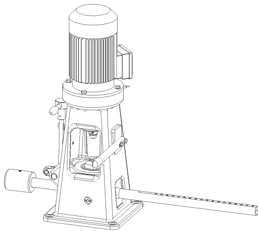
1 Stück Vierkugelapparat Grundgerät Motordrehzahl 1500\text{min}^{-1} 4-ball VKA 110 lubeoil tester - Engine speed 1500 rpm.
